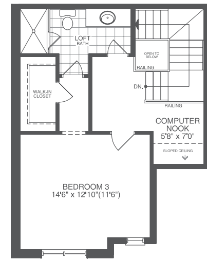
LOFT ELEV. A/B 1520/1518 sf
